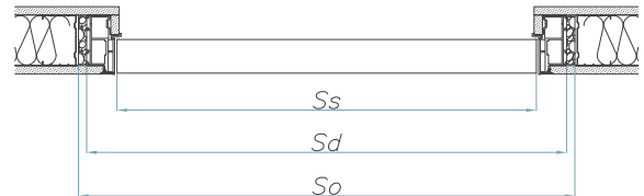
DRZWI OTWIERANE NA ZEWNĄTRZ ODZ
