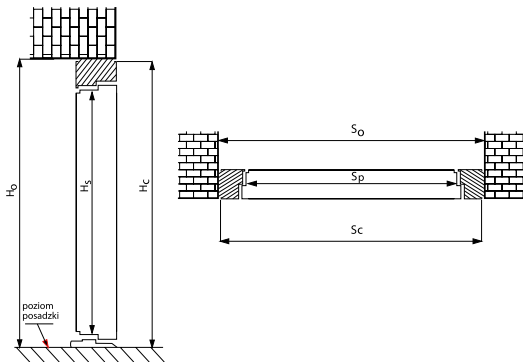
Wymiarowanie drzwi z ościeżnicą ALU HYBRID
