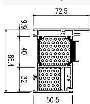
Rysunek techniczny
