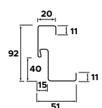
Rysunek techniczny
