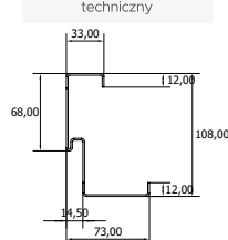
Rysunek techniczny
