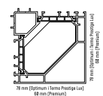
Rysunek techniczny
