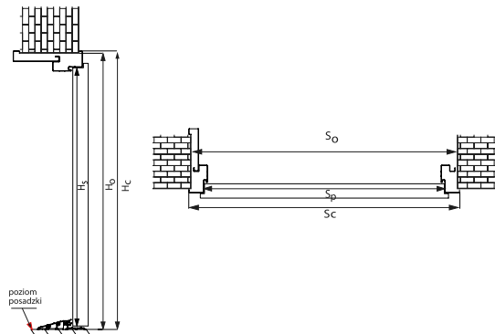
Wymiarowanie drzwi IRON z ościeżnicą symetryczną
