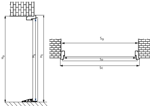
Wymiarowanie drzwi IRON z ościeżnicą kątową
