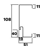
Rysunek techniczny
