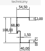
Rysunek techniczny
