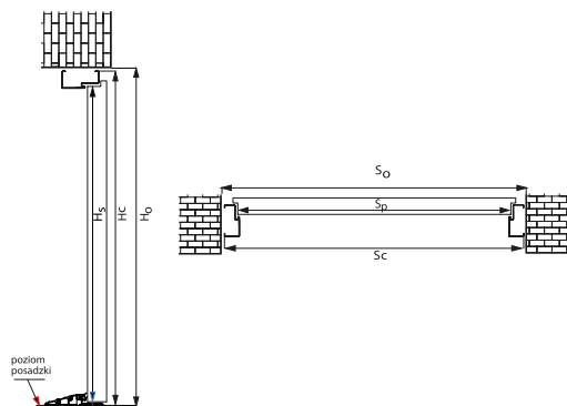
Wymiarowanie drzwi IRON z ościeżnicą symetryczną
