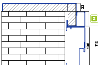
Ościeżnica Alu Hybrid
