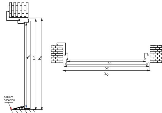
Wymiarowanie drzwi IRON z ościeżnicą wewnętrzną pod portal
