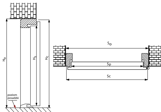
Wymiarowanie drzwi z ościeżnicą „11”, „12”, aluminiowo-kompozytową, drewniano-alumi- nową oraz TERMO i TERMO PRESTIGE LUX
