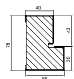
Rysunek techniczny
