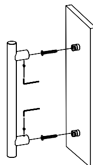
MONTAŻ POCHWYTU JEDNOSTRONNEGO NA DREWNOWKRĘT
