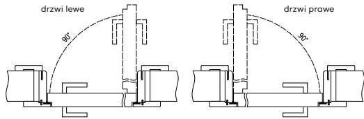
Profil ościeżnicy
