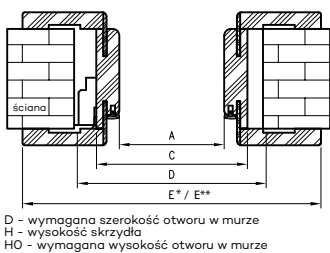
Przekrój OR z kątem T80
