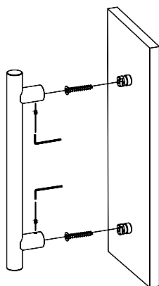
MONTAŻ POCHWYTU JEDNOSTRONNEGO NA DREWNOWKRĘT
