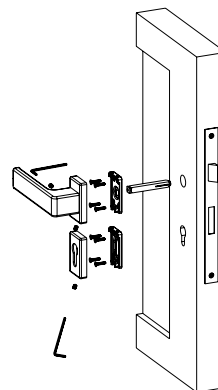
MONTAŻ KLAMKI NA ROZECIE Q11
