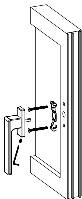
MONTAŻ KLAMKI OKIENNEJ I BALKONOWEJ
