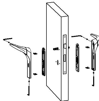
MONTAŻ KLAMKI MODEL 2055
