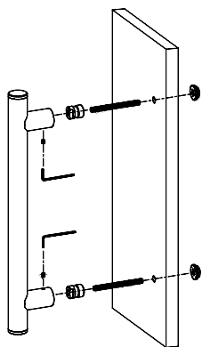
MONTAŻ POCHWYTU JEDNOSTRONNEGO NA PRZESTRZAŁ
