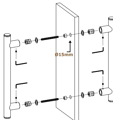
MONTAŻ POCHWYTU DWUSTRONNEGO DO DRZWI SZKLANYCH
