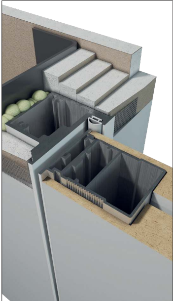
ZABUDOWA G-K - SKRZYDŁO Z RANTEM
