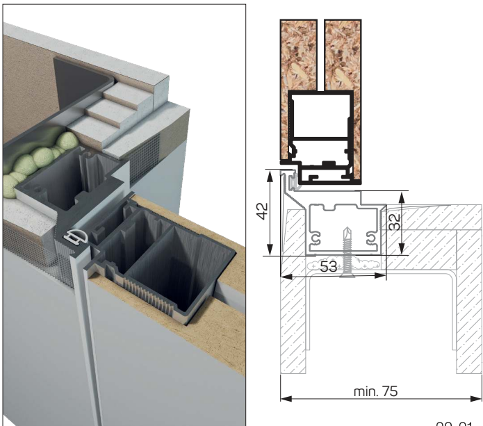
ZABUDOWA G-K - SKRZYDŁO Z RANTEM
