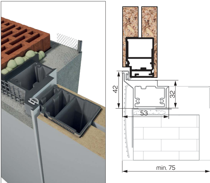
ZABUDOWA MUR - SKRZYDŁO BEZ RANTU
