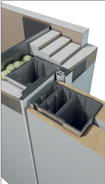
ZABUDOWA G-K - SKRZYDŁO BEZ RANTU
