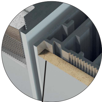
SKRZYDŁO Z RANTEM
