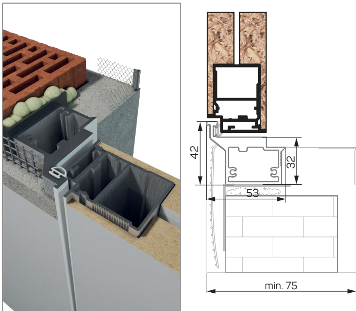
ZABUDOWA MUR - SKRZYDŁO Z RANTEM
