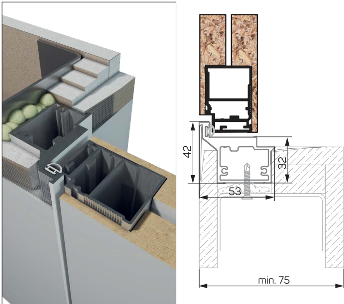
ZABUDOWA G-K - SKRZYDŁO BEZ RANTU
