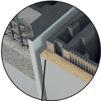
SKRZYDŁO BEZ RANTU
