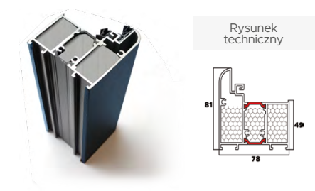
Ościeżnica "9" Premium / Normal
