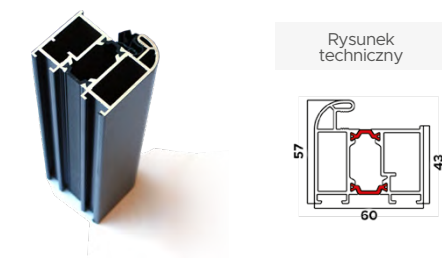
Ościeżnica "12" Optimum
