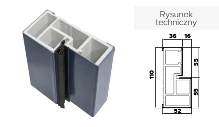
Ościeżnica aluminiowo-kompozytowa Optimum
