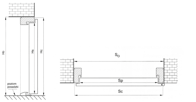
Wymiarowanie drzwi z ościeżnicą "11" , "12" , aluminiowo-kompozytową oraz TERMO i TERMO PRESTIGE
