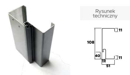
Ościeżnica "11" Premium / Normal
