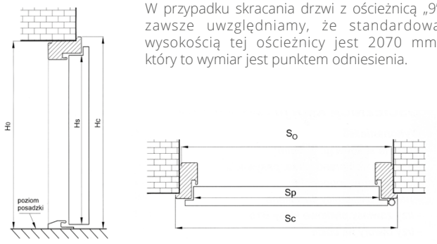
Wymiarowanie drzwi z ościeżnicą "9"
