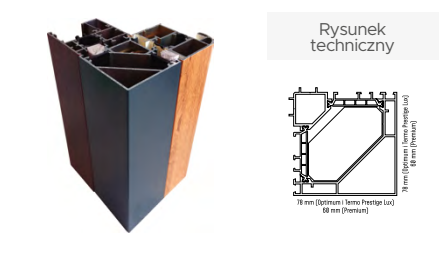
Przekrój łącznika kątownego Termo 90°
