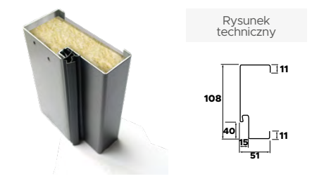
Ościeżnica "11" Protect
