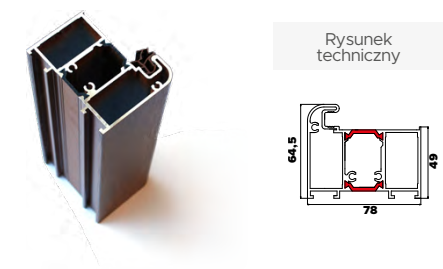
Ościeżnica "11" Premium / Normal
