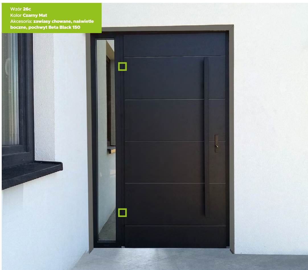
NIEWIDOCZNE Z ZEWNĄTRZ ZAWIASY CHOWANE
