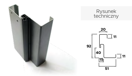
Ościeżnica "9" Premium / Normal
