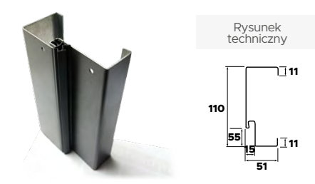
Ościeżnica "12" Optimum
