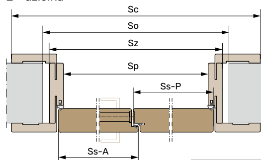
2 - dzielna
