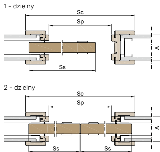
System wewnętrzścienny
